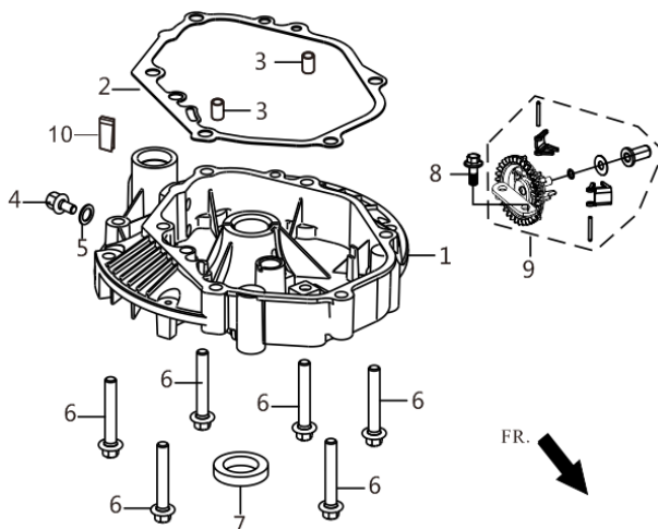
图3：曲轴箱盖部件 + 调速齿轮部件(E16)
