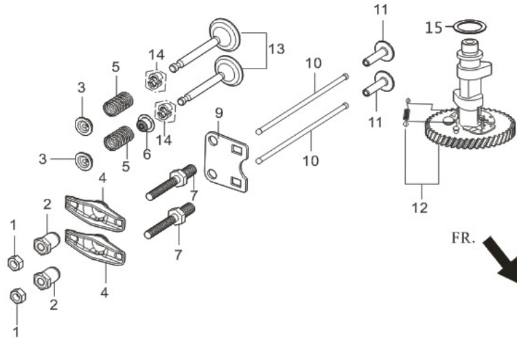
图5：配气机构组件/凸轮轴（E05）
