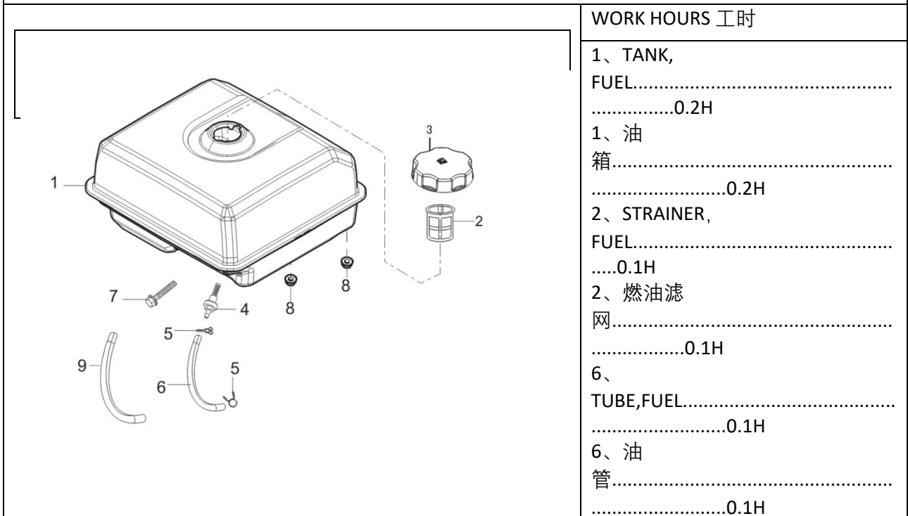
图 12 : 油箱部件 (F01)
